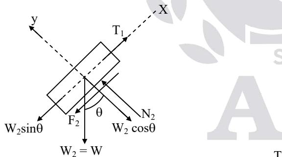
Fig: FBD (1)
